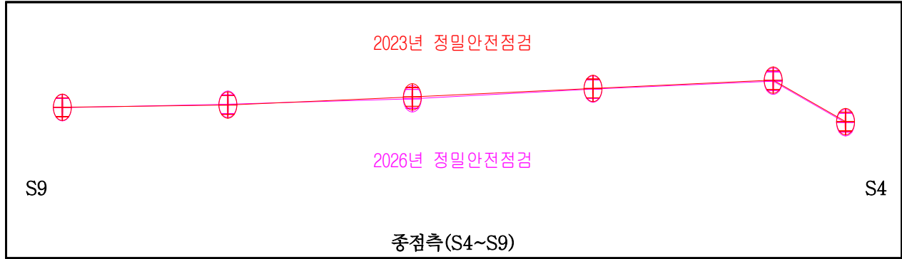
【그림 1.4.4】 수준측량(수직변위) 측정결과 비교(계속)
