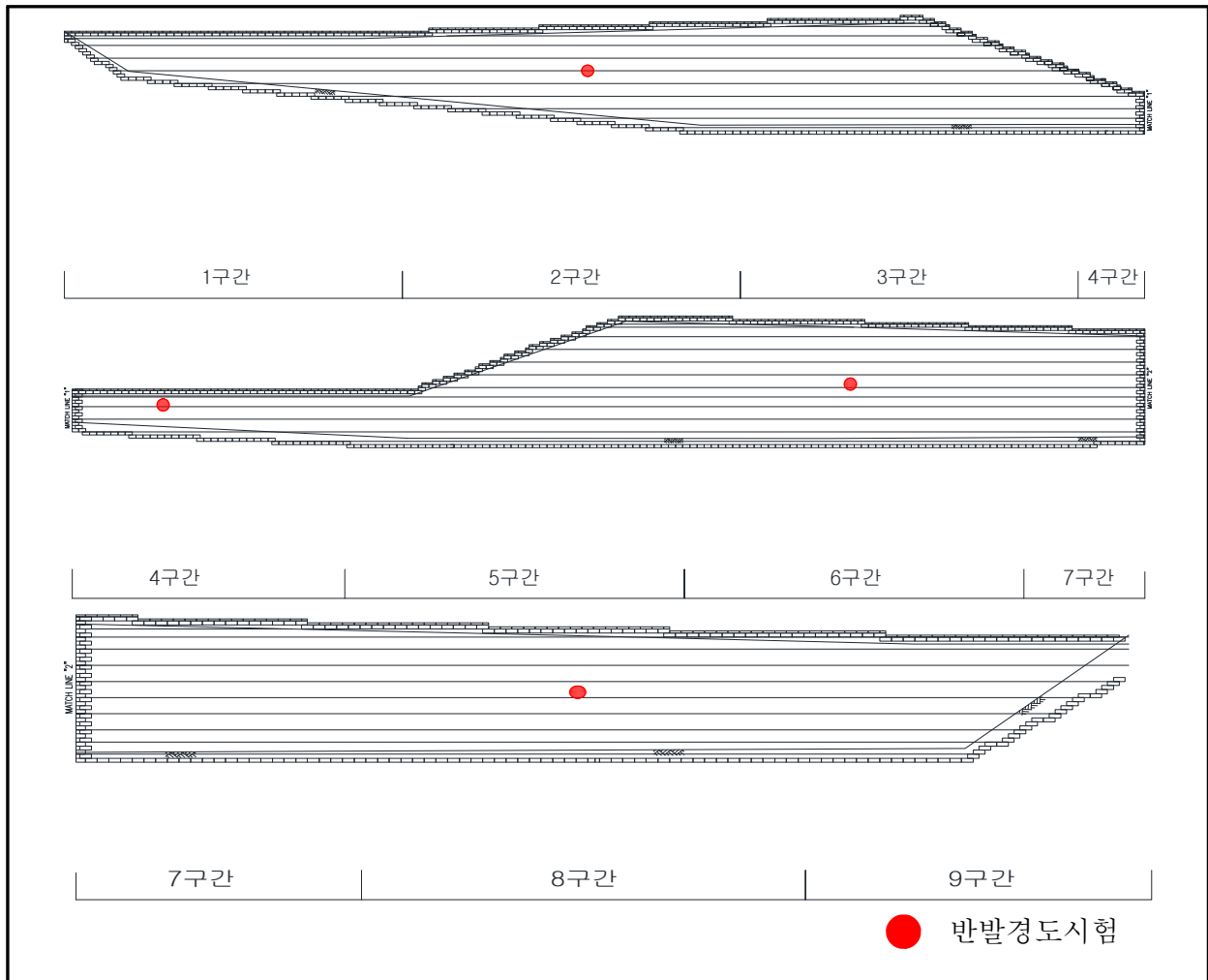
【그림 1.4.1】 콘크리트 재료시험 조사 위치도
