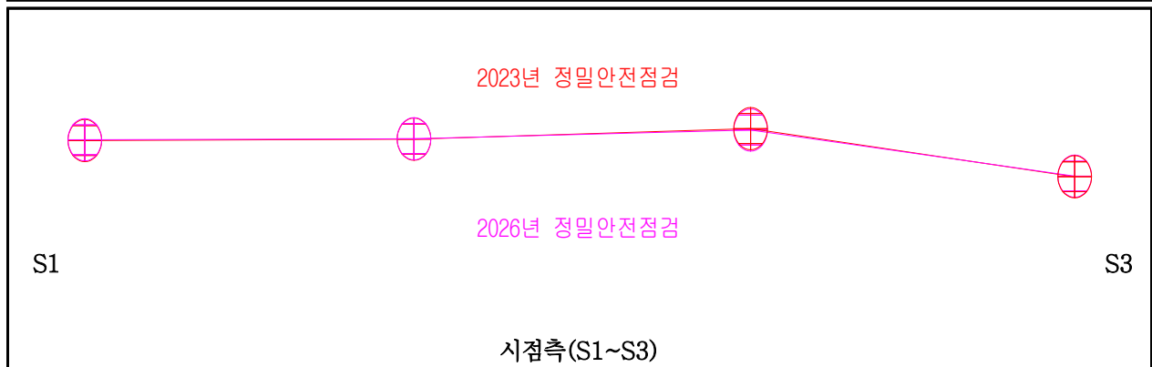
【그림 1.4.4】 수준측량(수직변위) 측정결과 비교
